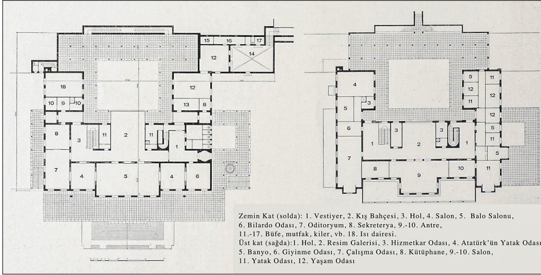
Şekil 4. Holzmeister tasarımı konutun plan çizimleri. Kaynak: Balamir, 2010, s. 358.
