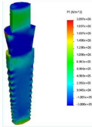
Şekil 19. Zirkonya abutment kullanılan modelde dikey kuvvet sonucu implant ve Ti-base'de oluşan maksimum asal gerilmeler
